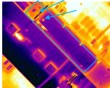
Avvik: kraftige varmesignaturer indikerer fukt i taket (NAS illustrasjonsfoto).
